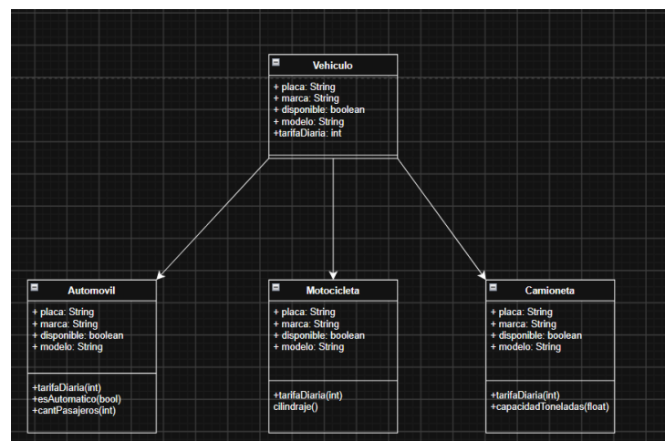
Diagrama UML
